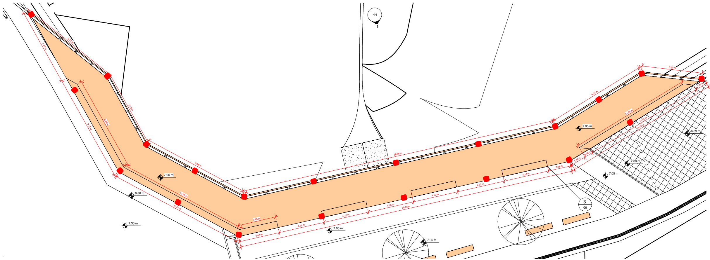
2 IDENTIFICAÇÃO BANCOS - DECK 1 : 100
