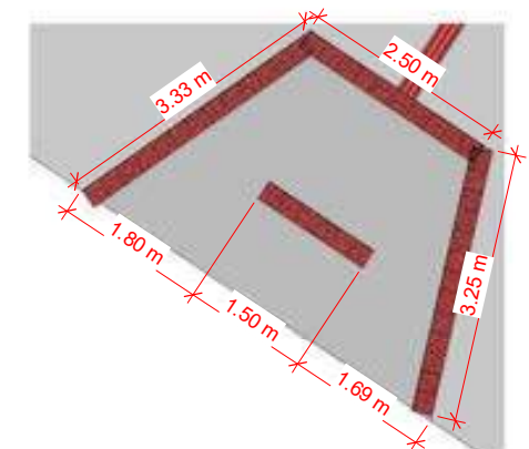
5 DETALHAMENTO RAMPA 1 : 50
