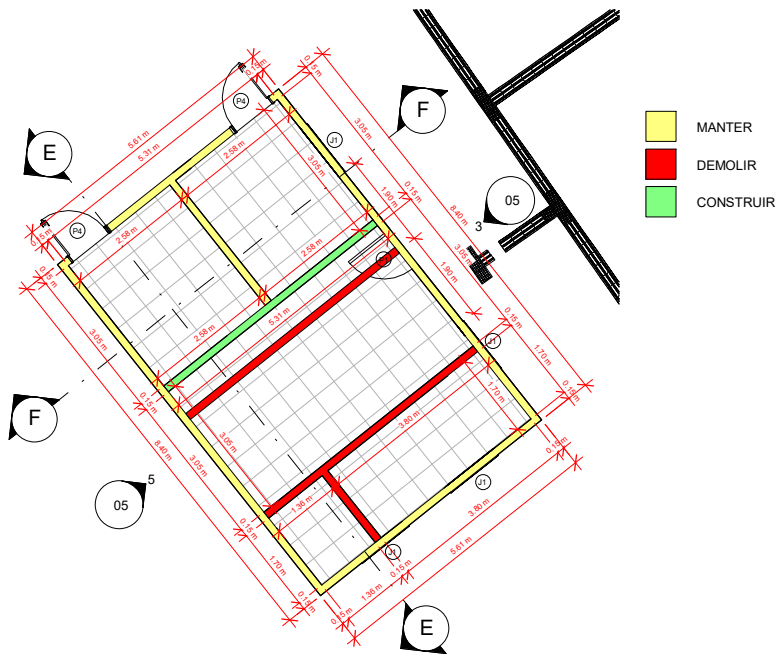
9 PLANTA BAIXA - DEMOLIR/CONSTRUIR 1 : 75
