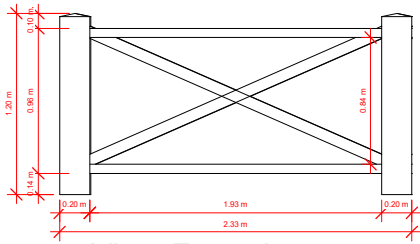
7 Vista Frontal 1 : 25
