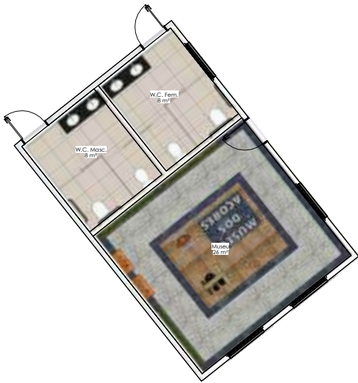
2 PREVISÃO DE AMBIENTAÇÃO PÓS REFORMA 1 : 75
