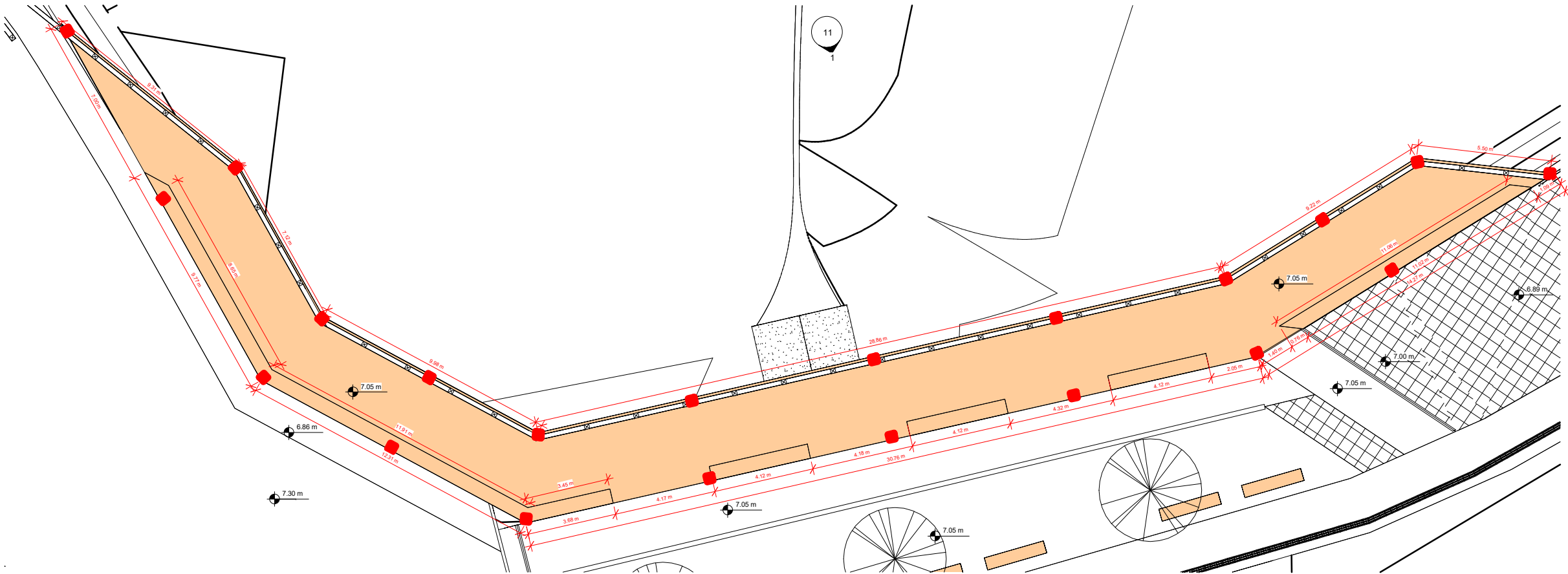
4 PLANTA BAIXA - DECK 1 : 100
