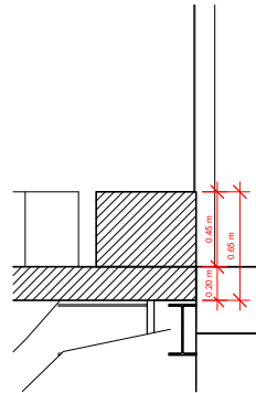
4 CORTE BANCO - DECK 1 : 25
