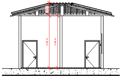
8 CORTE FF 1 : 75
