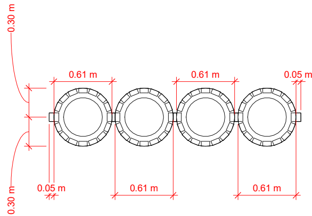
5 LIXEIRO 1 : 20
