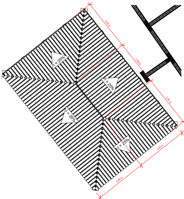
1 COBERTURA - QUIOSQUE 1 : 75
