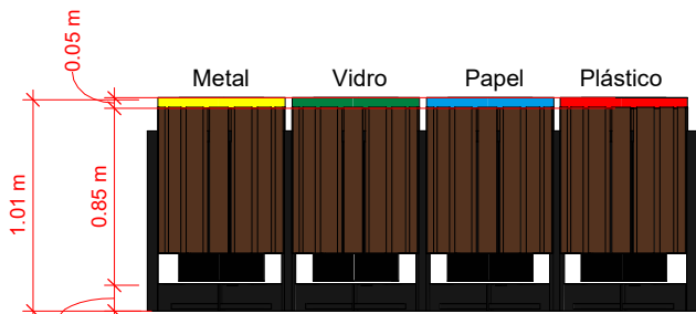
6 LIXEIRO -V1 1 : 20
