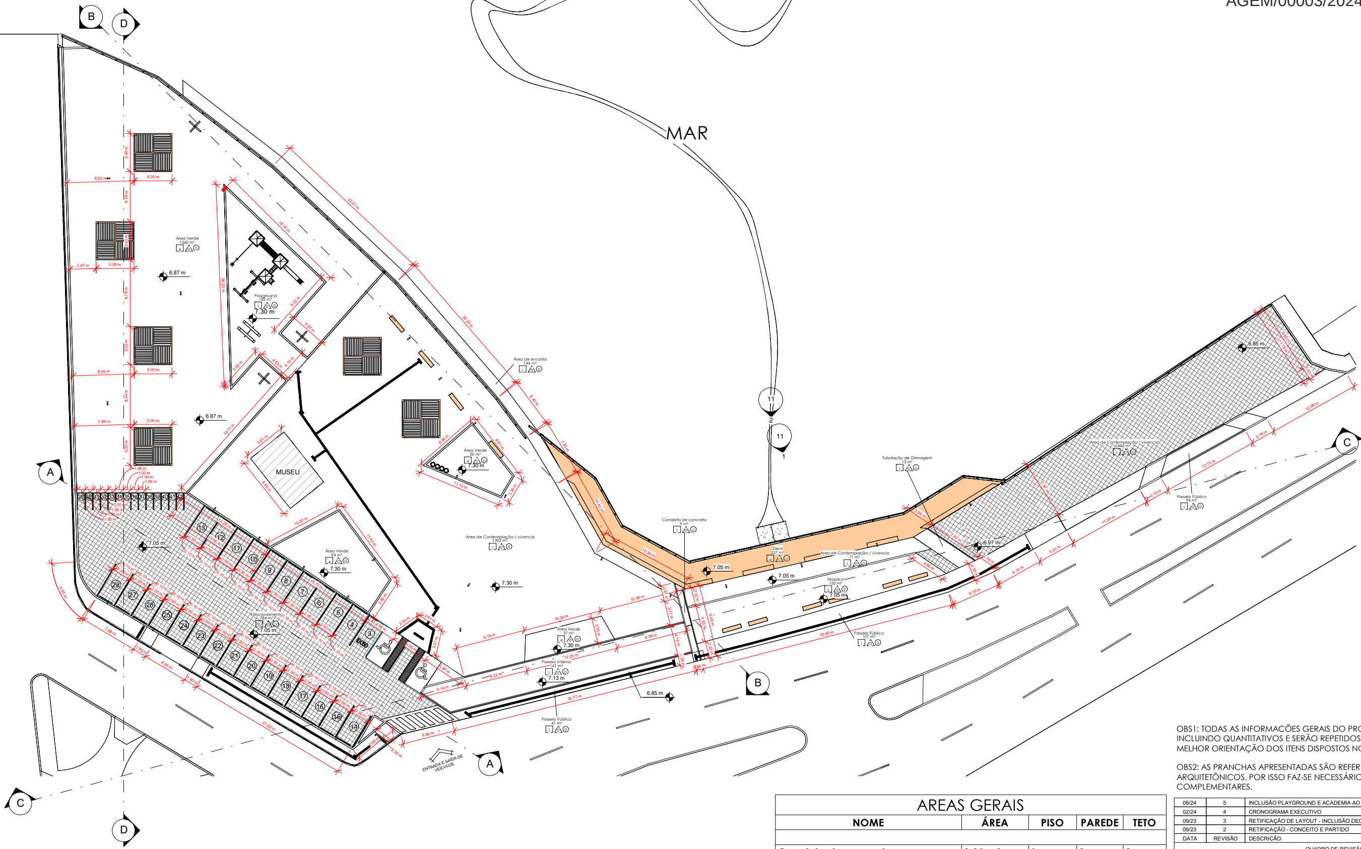
1 Planta Baixa 1 : 250
