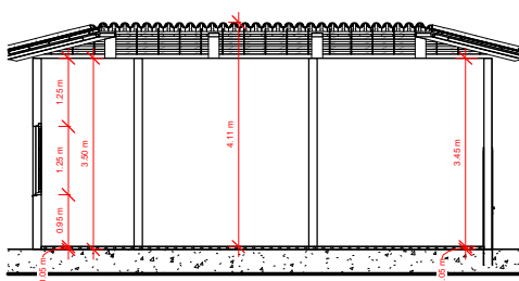
7 CORTE EE 1 : 75
